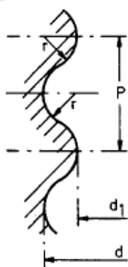
Detail of thread Détail du filetage
